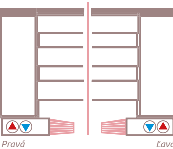
Nákres pripojenia Setu VHX-MONO.
